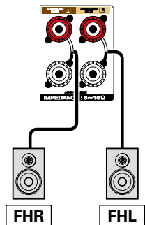
【フロントハイトスピーカーを接続する場合】
