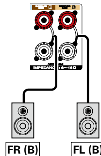
【フロントBスピーカーを接続する場合】
